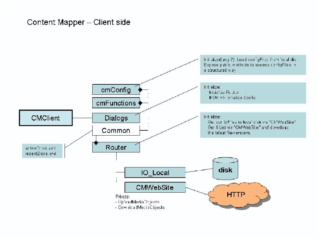
Figur 9.7: Kart over klientsiden av Content Mapper
