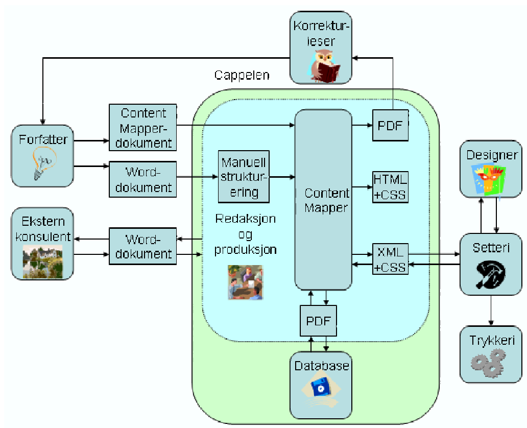
Figur 10.2: Forslag til ny manusflyt (detaljer) fortsettelse
