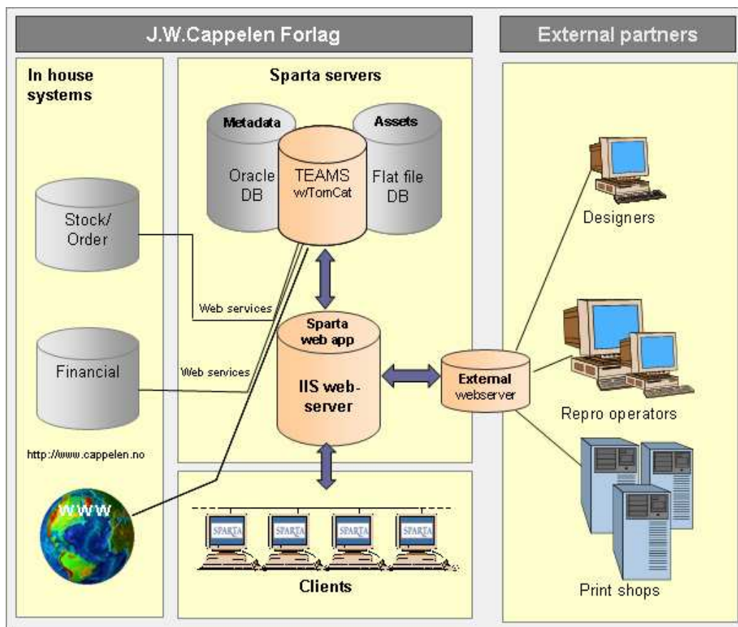
Figur 4.3: Sparta integrert i Cappelen
